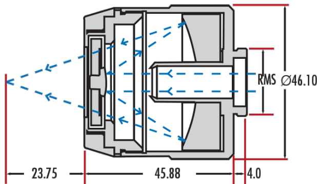
15X ReflX™ Objectives
